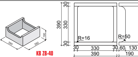
KB ZB-40
