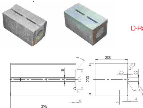
D-RainBlok zaústovací
