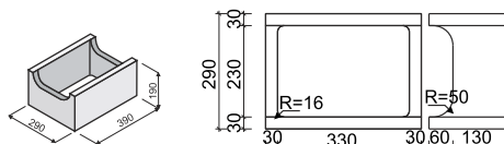
KB ZB-30
