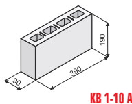
KB 1-10 A
