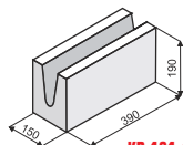
KB 101-15 A
