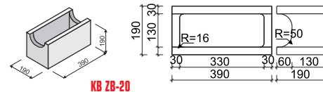
KB ZB-20
