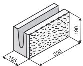
KB 101-15 B
