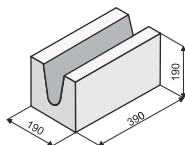
KB 101-20 A
