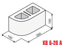
KB 6-20 A
